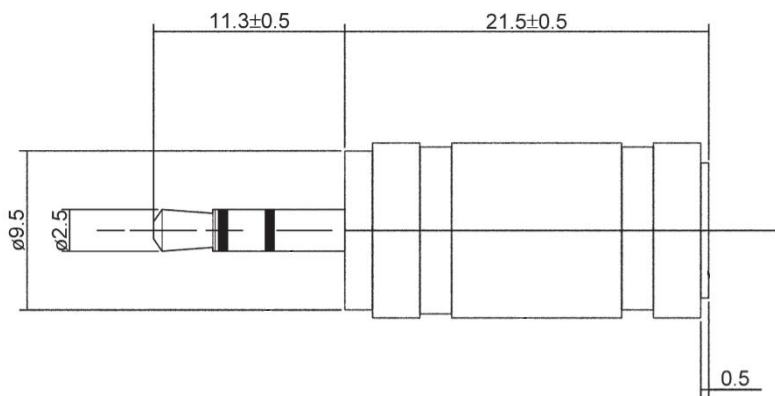
штекер 2,5мм стерео
