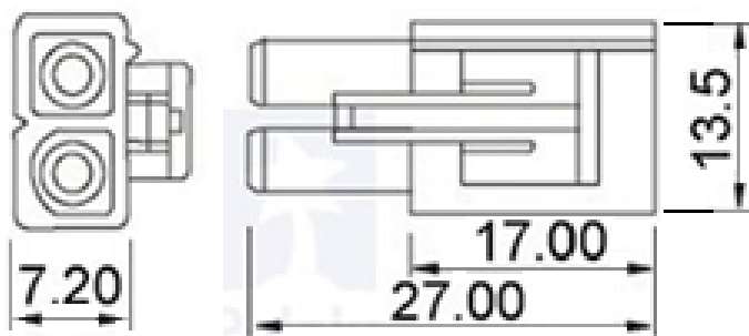
штекер MFA [Tamiya M]
