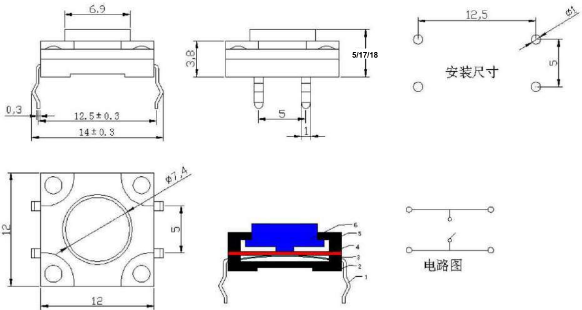
尺寸外型图
