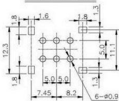
P.C.B HOLE DETAIL
