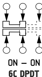
Схема работы переключателя
