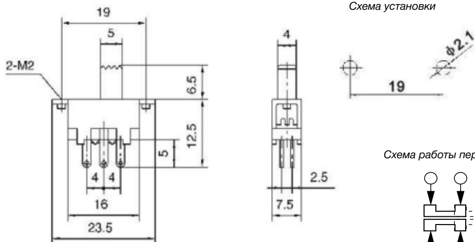
Схема установки
