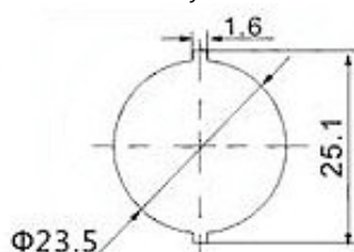
Схема установки
