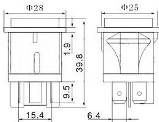
Схема установки
