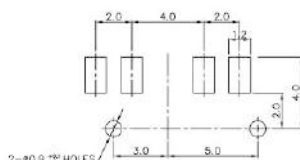
Схема установки
