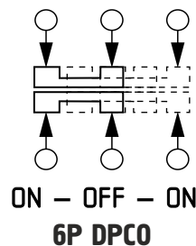
Схема работы переключателя
