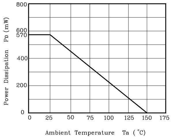
Fig. 4 P_D-T_a
