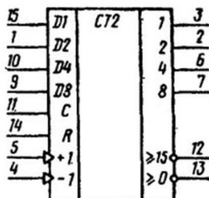
Условное графическое изображение K155IE7, KM155IE7
