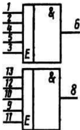
Условное графическое обозначение К511ЛИ1
