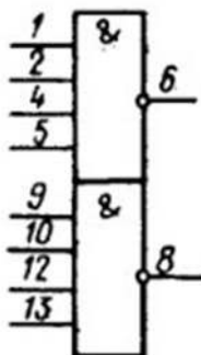
Условное графическое обозначение К155ЛА1, КМ155ЛА1, КБ155ЛА1-4
