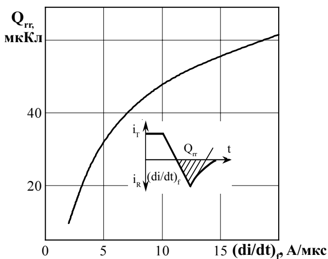
Рисунок 17 - Зависимость заряда восстановления Q_{rr} от скорости спада тока (di/dt)_f в открытом состоянии при температуре перехода T_{jm} = 125\text{ }^\circ\text{C} , U_{RM} = 100\text{ В} ; I_T = I_{T(AV)} .
