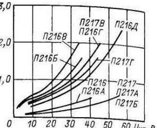
Зависимость обратного тока коллектора от напряжения коллектор-база.
