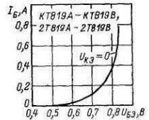
Входная характеристика.
