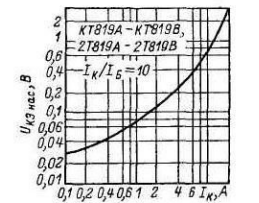
Зависимость напряжения насыщения коллектор-эмиттер от тока коллектора.
