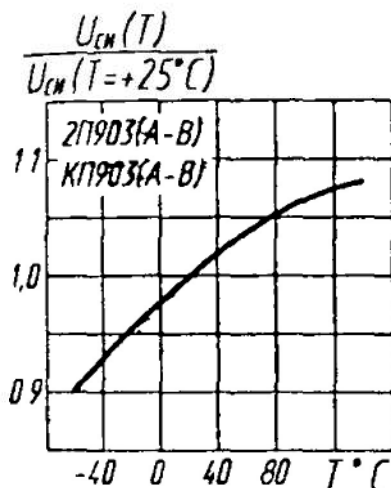
Зависимость относительного изменения пробивного напряжения сток—исток от температуры
