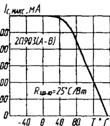
Зависимость допустимого тока стока от температуры
