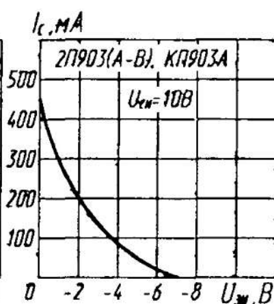
Зависимость тока стока от напряжения затвор—исток
