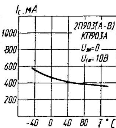
Зависимость тока стока от температуры
