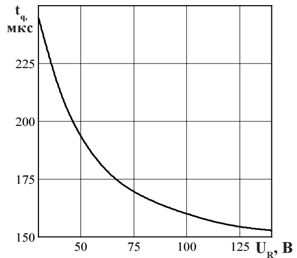
Рисунок 15 - Зависимость времени выключения t_q от обратного напряжения U_R при максимальной температуре перехода T_{jm} = 100^\circ C ; I_T = I_{TAVM} ; (di/dt)_f = 5 A/мкс ; dU_D/dt = 50 В/мкс ; U_D = 0,67 U_{DRM}
