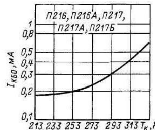
Зависимость обратного тока коллектора от температуры корпуса.
