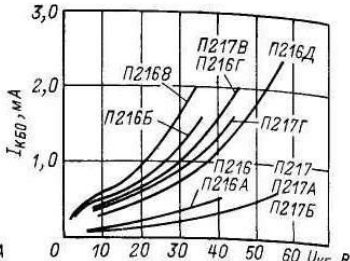
Зависимость обратного тока коллектора от напряжения коллектор-база.
