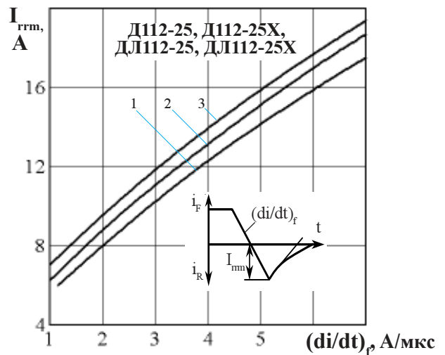
Рисунок 16 - Зависимость обратного тока восстановления I_{rrm} от скорости спада прямого тока (di/dt)_f при температуре перехода T_{jm} = 150^\circ\text{C} , U_R = 100\text{ В} и при отношении амплитуды прямого тока I_F к допустимому среднему прямому току I_{F(AV)} равному: k = 0,5 (1); 1,0 (2); 1,5 (3); где k = I_F/I_{F(AV)} .
