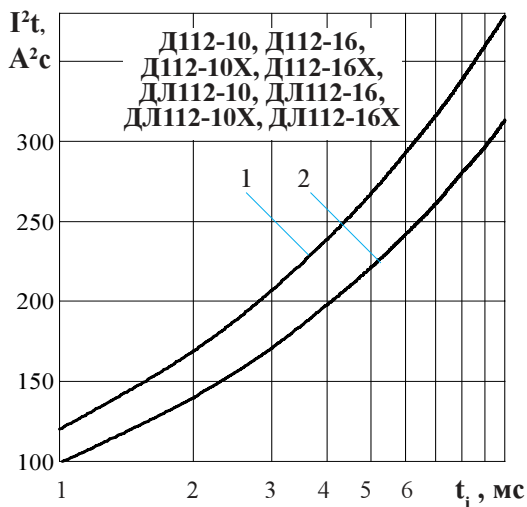
Рисунок 9 - Зависимость защитного показателя \Gamma^t от длительности импульса тока t_i при исходной температуре структуры T_j = 25 °C (1) и максимальной температуре T_{jm} (2)
