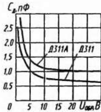
Зависимости общей емкости диода от напряжения
