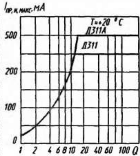
Зависимости максимального импульсного прямого тока от скажности
