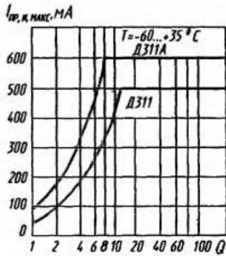
Зависимости максимального импульсного прямого тока от скажности
