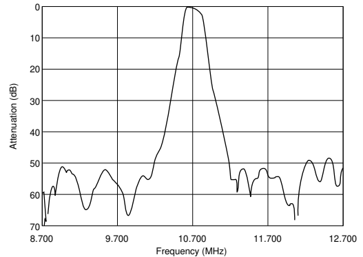
SFELA10M7GA00-B0
