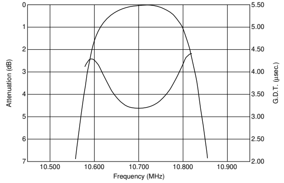
SFECV10M7GA00-R0
