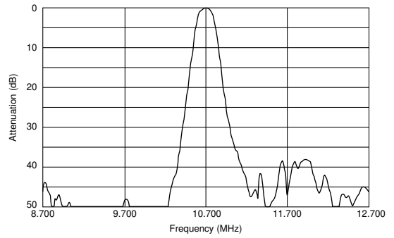
SFECS10M7GA00-R0
