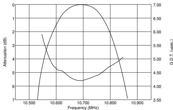
SFTLA10M7GA00-B0
