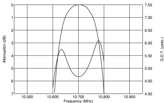
SFELA10M7JAA0-B0
