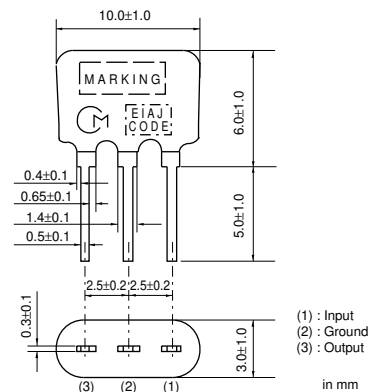
SFTLA10M7FA00-B0
