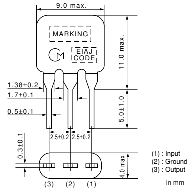
SFELA10M7GAXX-B0
