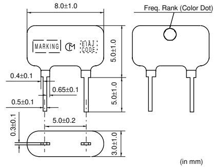
CDALA10M7G_Series
