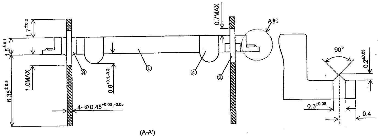
A部详图(20:1)
