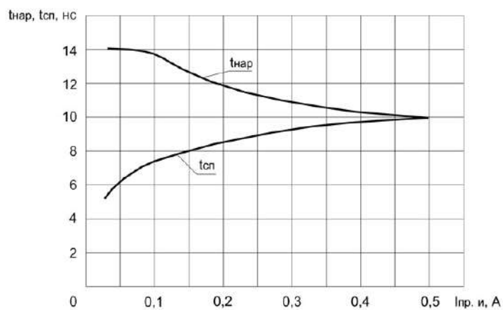
Зависимость времени нарастания и спада импульса излучения от прямого импульсного тока при T_{кр} = (25 \pm 10) \text{ } ^\circ\text{C}
