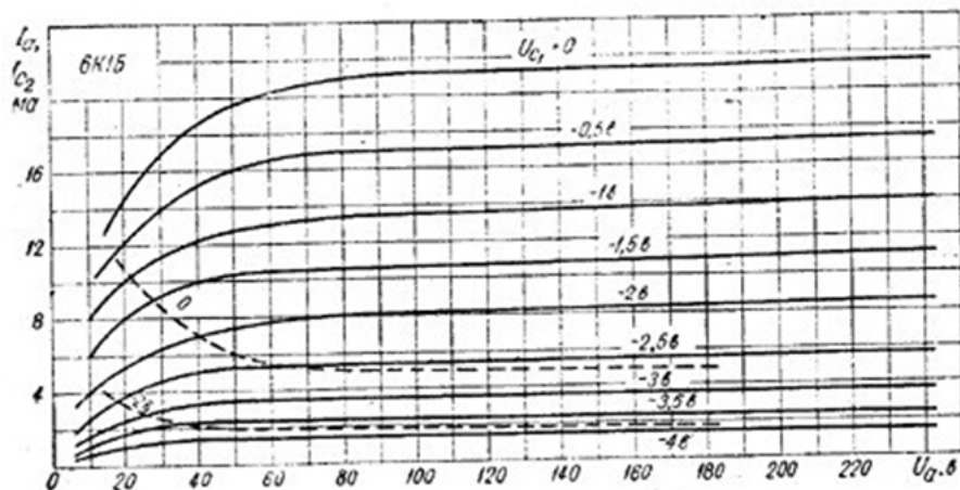
Рис. 238. Усредненные характеристики зависимости тока анода и тока второй сетки от напряжения на аноде при напряжении на второй сетке 120 в: — ток в цепи анода; — — — ток в цепи второй сетки.
