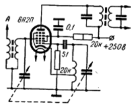
Рис. 143. Схема применения лампы 6А2П в качестве преобразователя с гетеродином, выполненным по трехточечной схеме.
