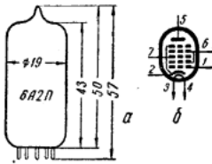
Рис. 139. Лампа 6А2П: а — основные размеры; б — схематическое изображение; 1 — первая сетка; 2 — накал и пятая сетка; 3 и 4 — подогреватель (накал); 5 — анод; 6 — вторая и четвертая сетки; 7 — третья сетка (сигнальная).
