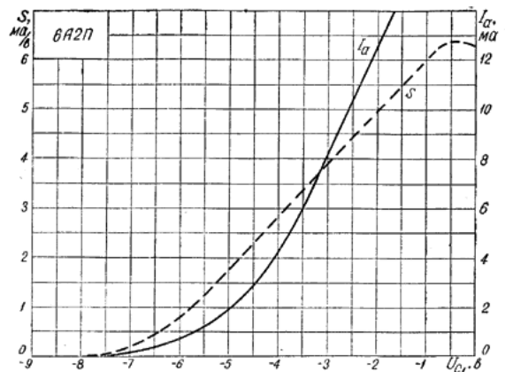
Рис. 142. Усредненные характеристики зависимости тока анода и крутизны гетеродина от напряжения на первой сетке при напряжении на аноде, второй и четвертой сетках 100 в, напряжении на третьей сетке 0: — ток в цепи анода; — — крутизна характеристики.
