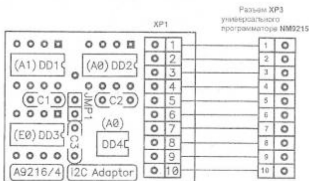
Рис.2 Монтажная схема
