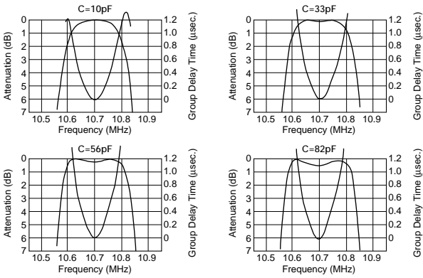
SFELA10M7GA00-B0
