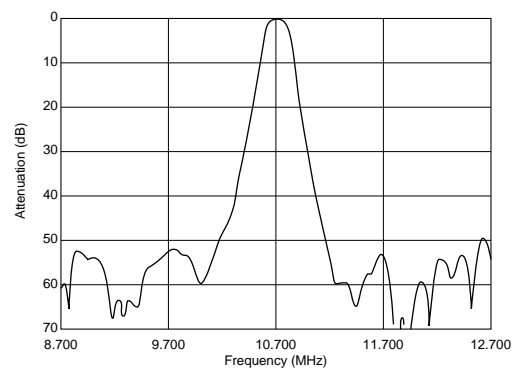
SFELB10M7GA00-B0
