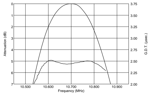
SFELA10M7GAXA-B0
