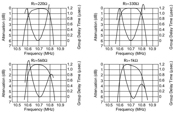
SFELA10M7GA00-B0
