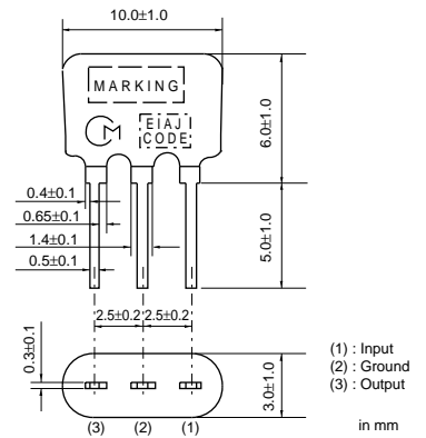
SFTLA10M7FA00-B0
